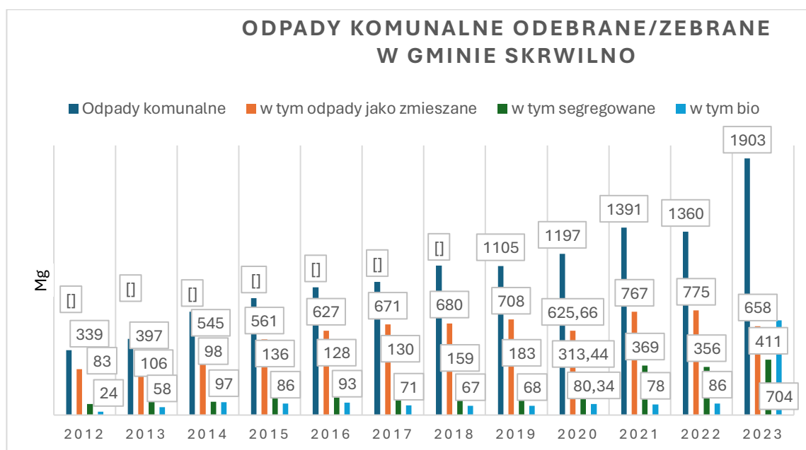
Rys. 1. Odpady komunalne odebrane/zebrane w Gminie Skrwilno w latach 2012-2023, Mg
