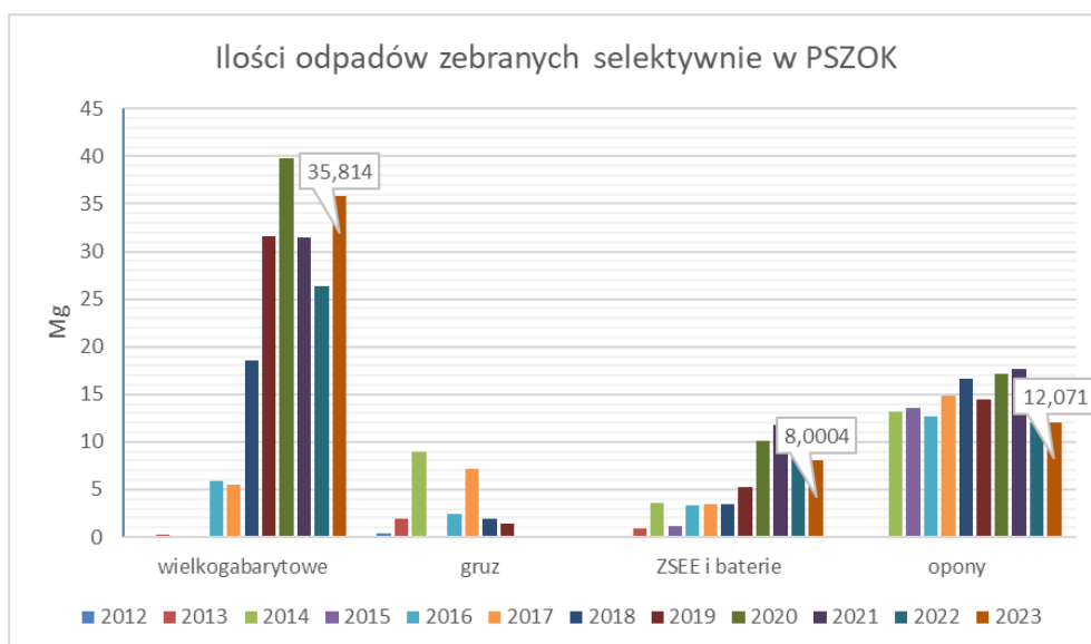
Rys. 3. Ilości selektywnie zebranych odpadów wielkogabarytowych, budowlanych, ZSEE i baterii i opon łącznie w latach 2012 – 2023, Mg
